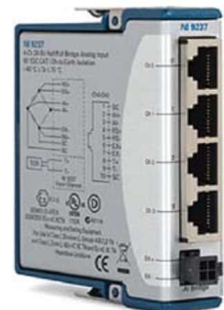
Brückenmodul mit simultaner Abtastung
